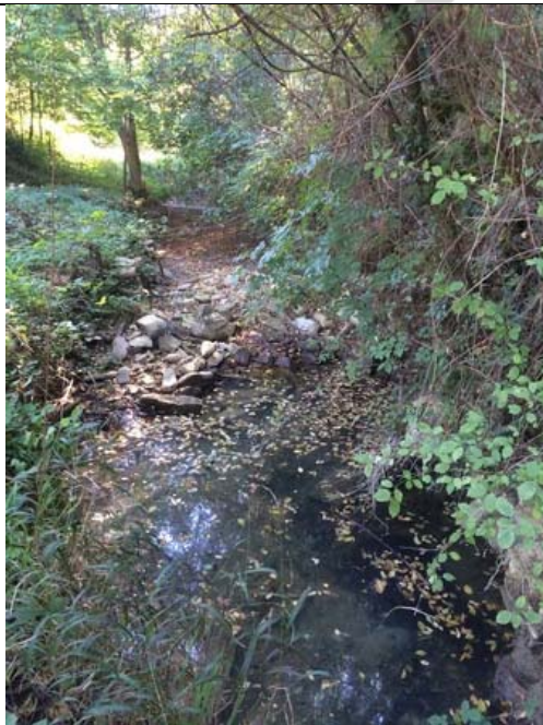
Slika 5: Kosi peščenjaka in laporovca v strugi potoka – lokacija Korte
